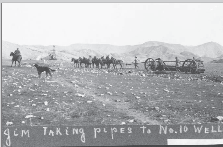
حمل لوله نفت بوسیله چهارپایان برای چاه شماره ۱۰
